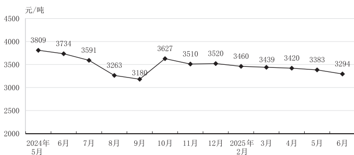
钢坯（管坯）价格走势
